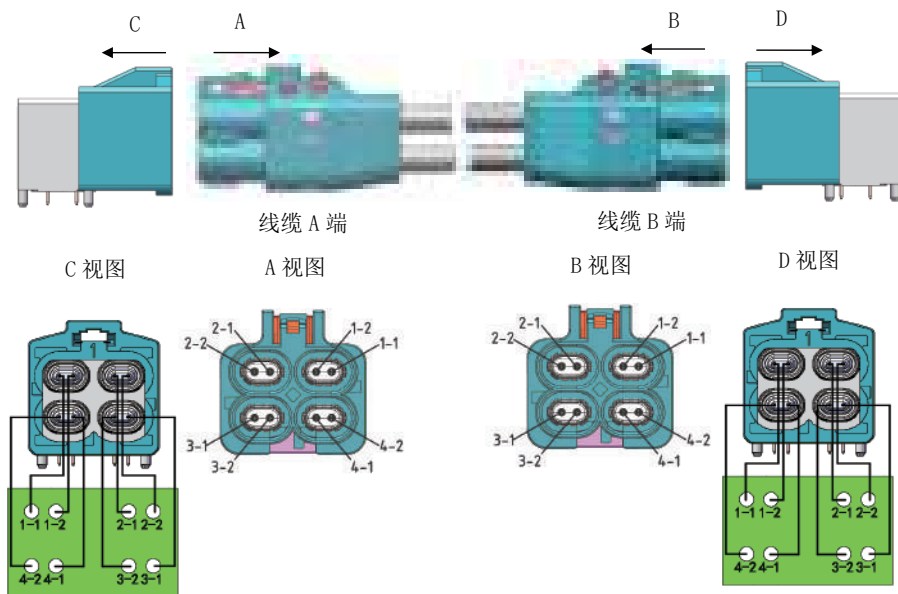
【4Pair线缆组件(带CPA)】
