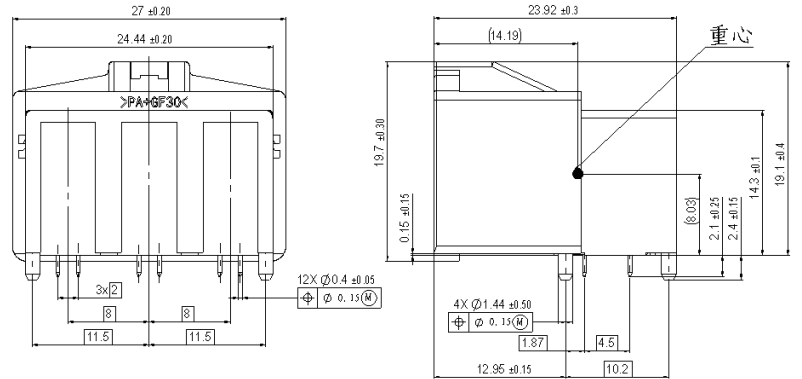
6Pair板端外形尺寸
