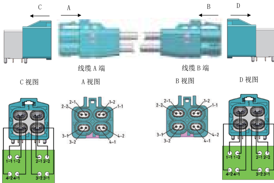
【4Pair线缆组件(不带CPA)】
