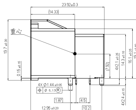
4Pair板端外形尺寸
