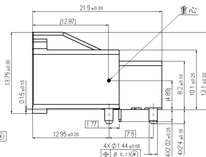
2Pair板端外形尺寸
