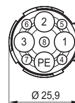
Розеточная часть M3 E-8S+PE
