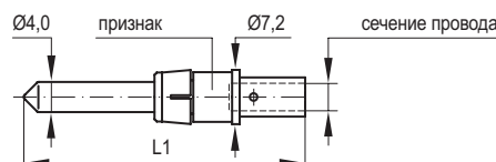
Штырьевой контакт, покрытие: серебро
