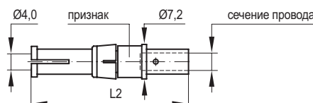
Гнездовой контакт, покрытие: серебро
