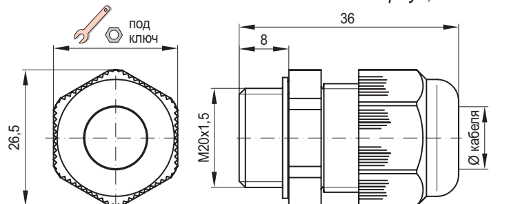
Корпус, часть 2
