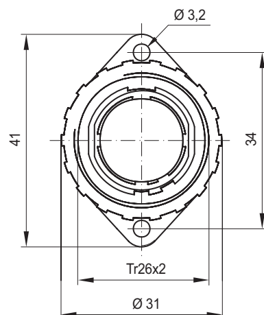
Корпус, часть 1
