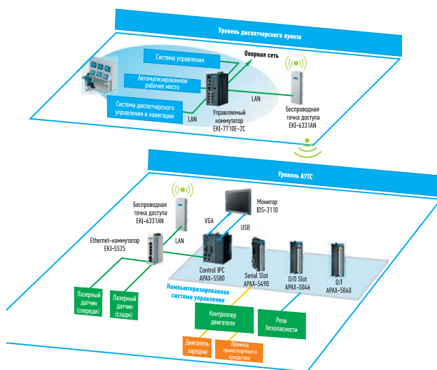
Рис. 2. Структура системы на основе компьютеризированного ПЛК
